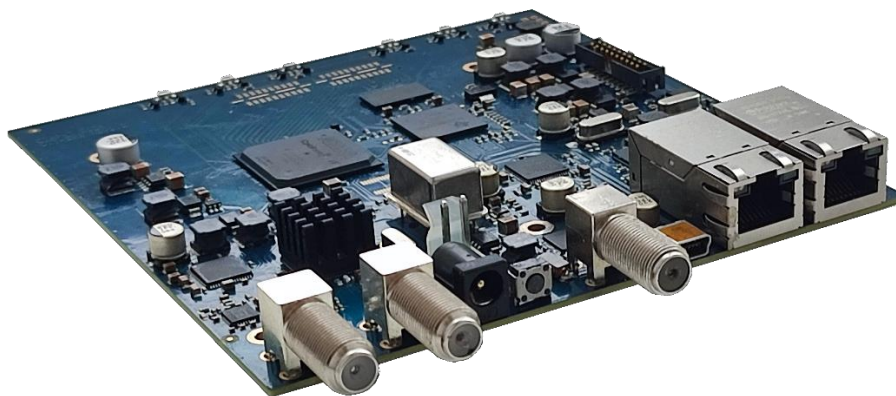
Рисунок 1. Внешний вид спутникового маршрутизатора СТТ-210
