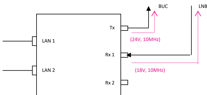
Рисунок 8. Схема стандартного подключения маршрутизатора СТТ-210
