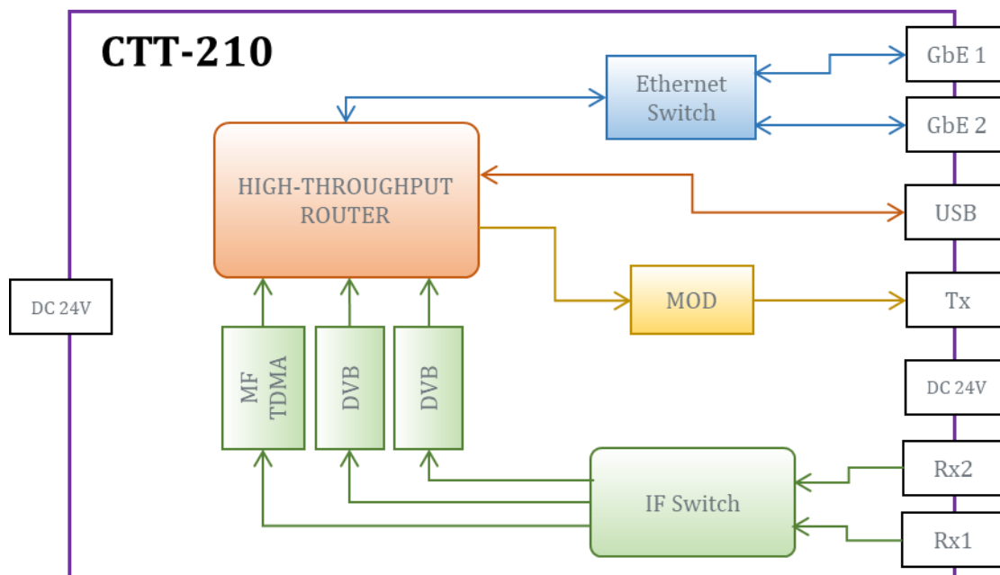
Рисунок 5. Структурная схема маршрутизатора СТТ-210
